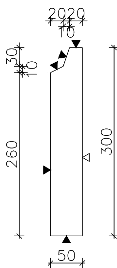
Doorsnede
