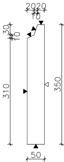
Doorsnede
