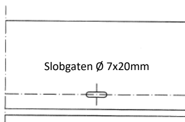
Gaten in hoeklijn GD of LA
